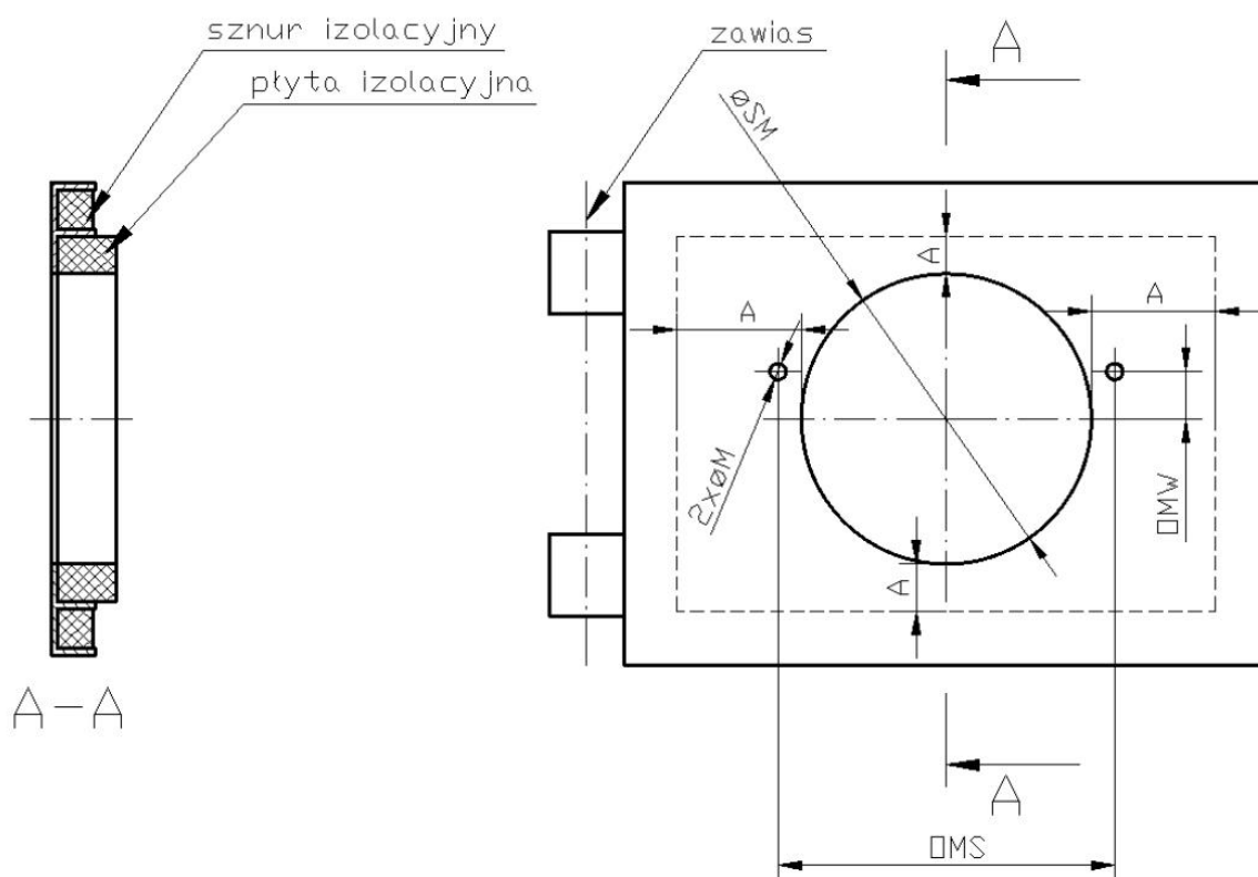
Rys. 3. Schemat wykonania otworów montażowych dla palników: 15-70 kW, 20-100 kW.
