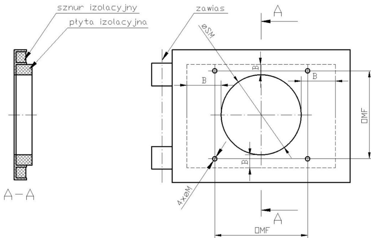
Rys. 4. Schemat wykonania otworów montażowych dla palnika z płaszczem izolacyjnym i płytą montażową dla palników: 15-70 kW, 20-100 kW.
