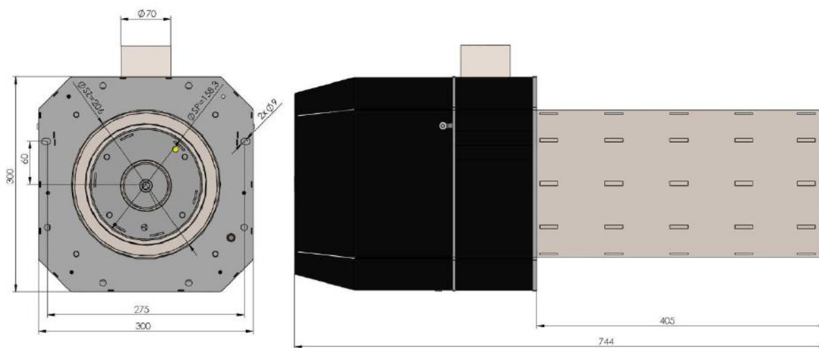
Rys. 19. Widok palnika 20-100 kW.
