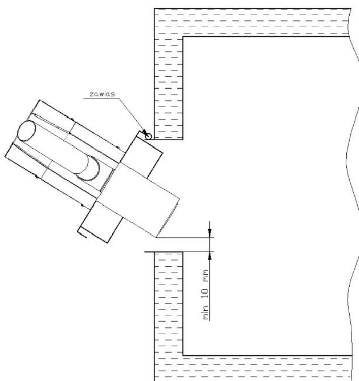
Rys. 5. Widok komory paleniska kotła w przekroju z góry.
