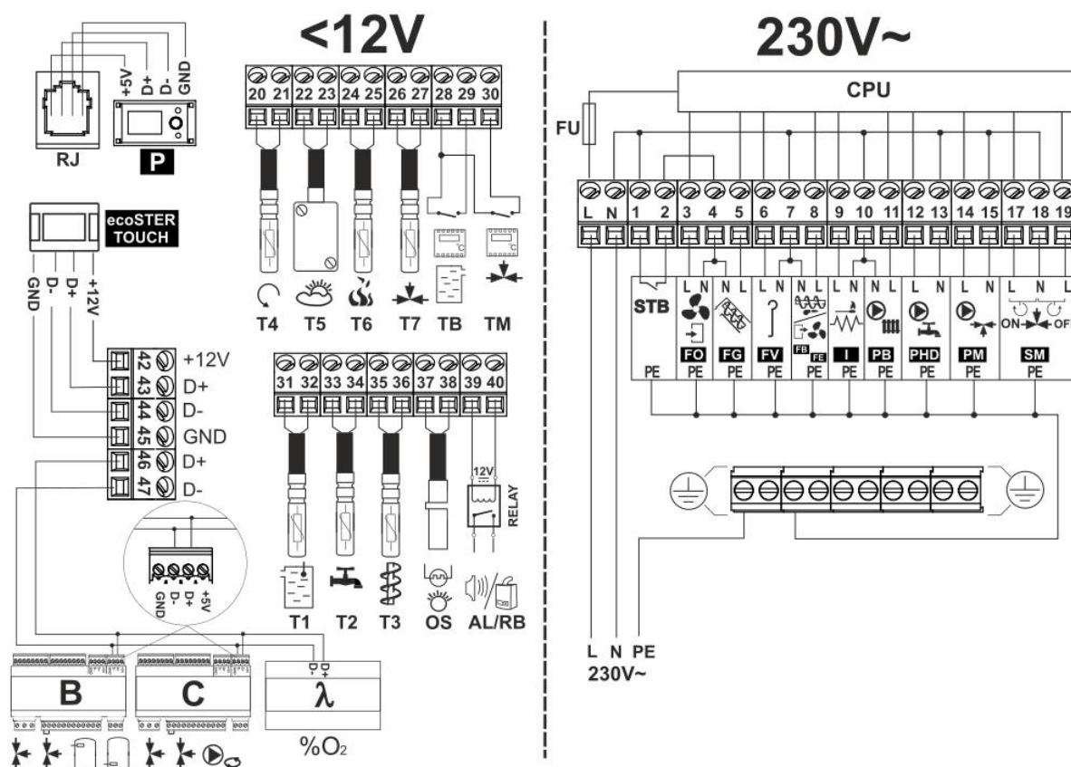
Rys. 13. Schemat połączeń elektrycznych regulatorów ecoMAX 850P ecoTOUCH 850P.
