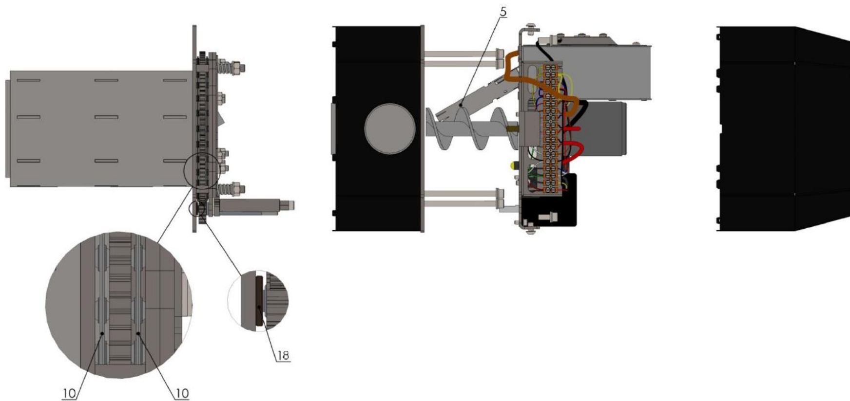
Rys. 11. Smarowanie łożysk komory spalania – widok 2.
