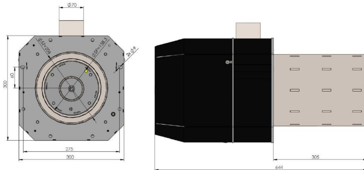
Rys. 17. Widok palnika 15-70 kW.
