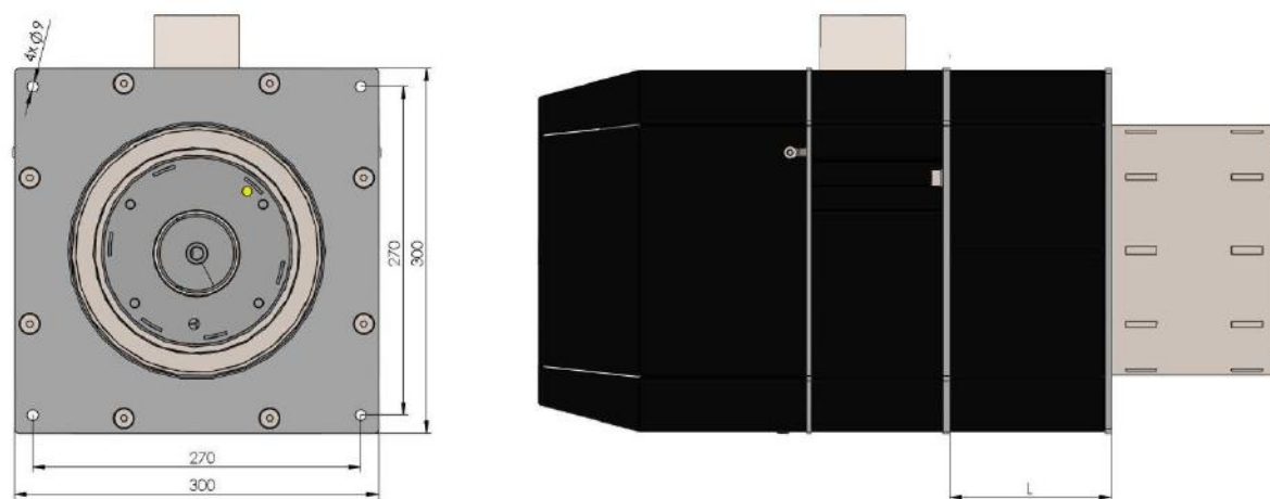
Rys. 17. Widok palnika 15-70 kW.
