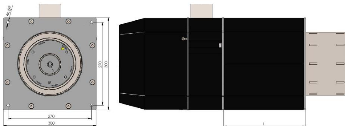
Rys. 20. Widok palnika 20-100 kW z płaszczem izolacyjnym i płytą montażową.
